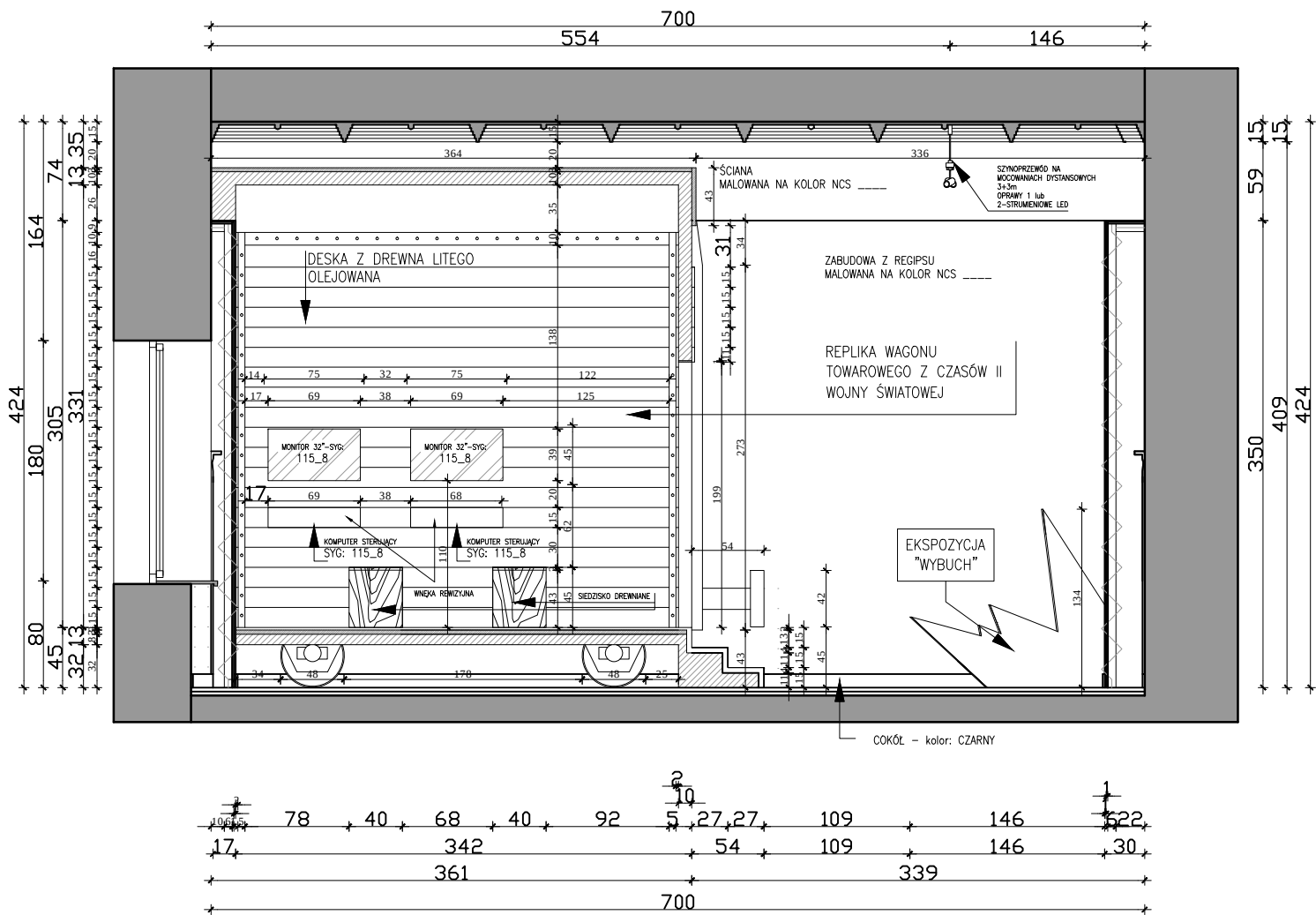
PRZEKROJ A6-A6 POM. NR 115
