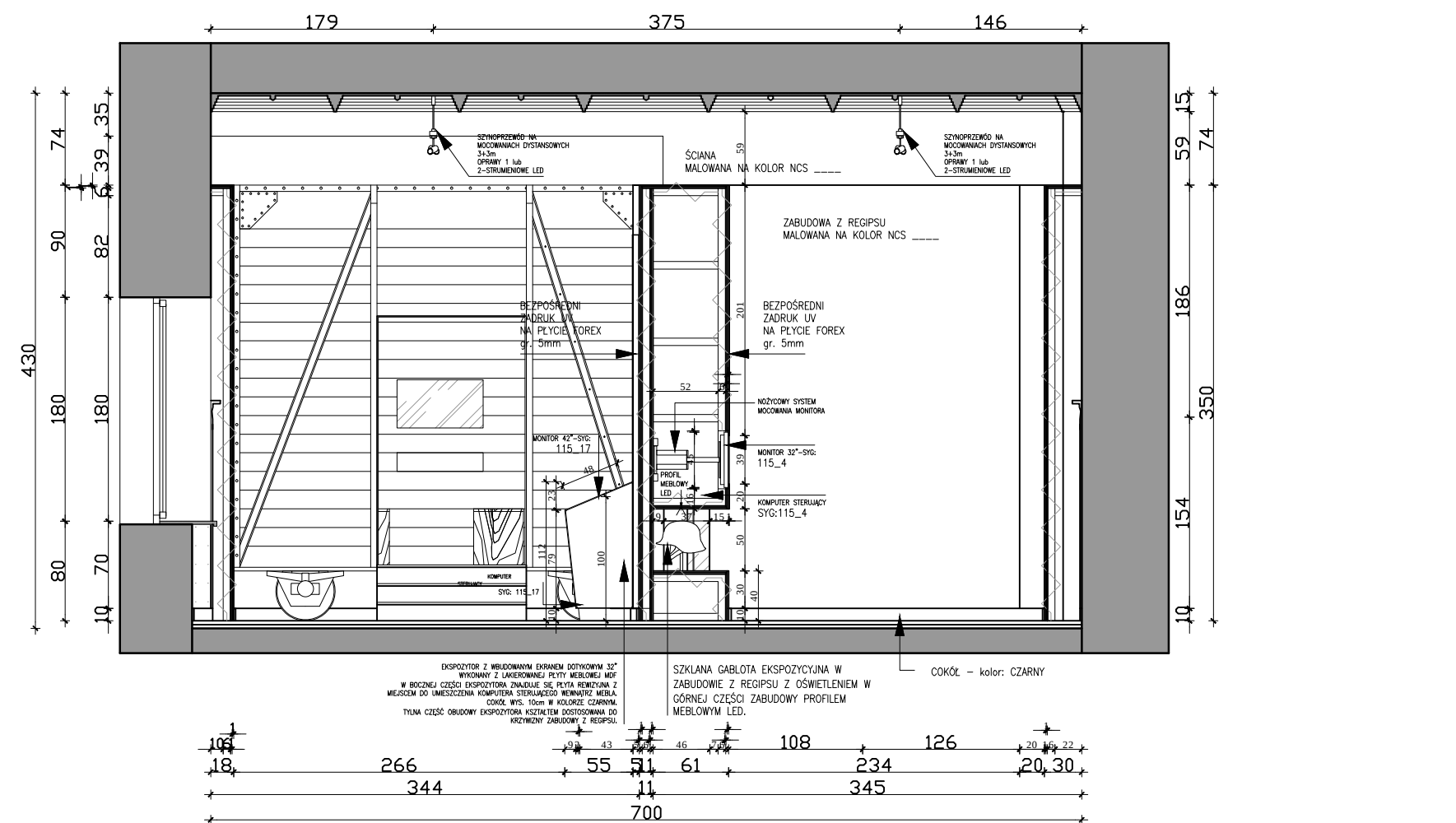
SCHEMAT LOKALIZACJI OPRAWY POMIESZCZENIOWYCH
